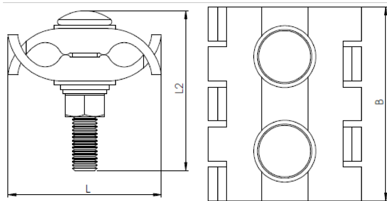
کلمپ جمپر مقطع 70 و 120
