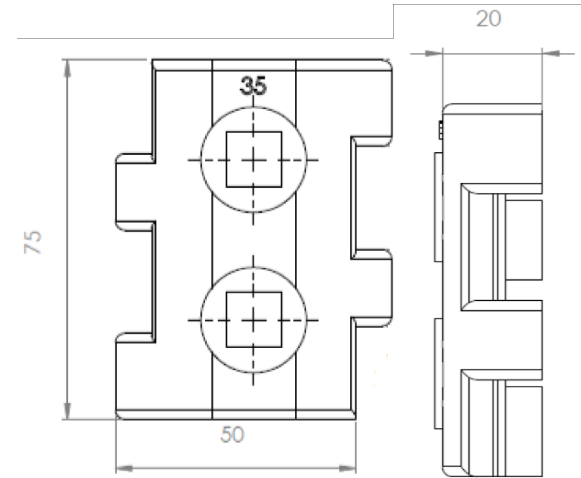
کلمپ جمپر مقطع 35
